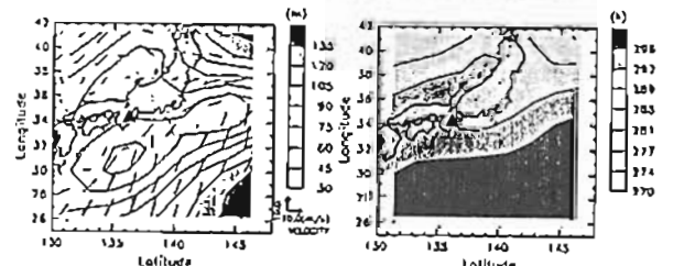
図 2: 6 月 18 日 0 時の 1000 hPa の気圧 (左) と温度 (右)。(▲ は観測地点の位置)
