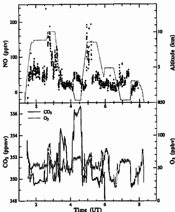
上図 台湾近海で観測されたNOの濃度比(点線)と観測機の飛行高度(点線) 下図 同時に観測されたCO 2 (実線)とO 3 (点線)の濃度比
