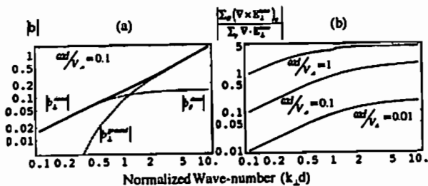
(a): 地上磁場の経度効果と、(b): 磁力線電位のHall部分とPedersen部分との比に対する水平方向の放射依存性 伝導度は \Sigma_A=1 , \Sigma_p=5 , \Sigma_m=10 に固定
