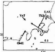
図1 インダクションベクトルの変化分 (1989年7月~8月)
