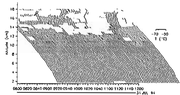
図1: 1994年7月31日0800LT~1200LTにMUレーダー/RASSにより103秒間隔で観測された仮温度の高度プロファイル。
