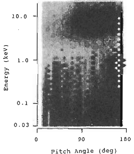
図1. Suprathermal electron burstsのエネルギー・ビッチ角分布の例。最も活発なバーストの多いことを示す。20秒間のデータの1秒分で、この観測時間1~2秒のバーストが観測されている。
