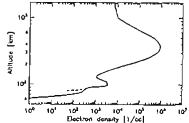
図 2: 計算に用いた電子密度プロファイル
