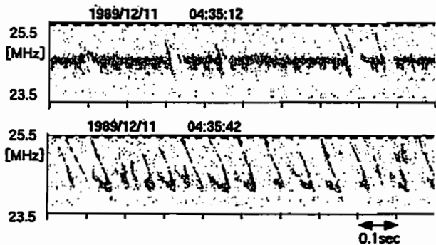
図 1: 1989 年 12 月 11 日に観測された S パースト (上部の黒いマークは右旋偏波を示す)
