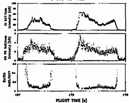
図2. 図1と同じ時間帯でのOI 557.7nm線とN 2 VK 342.5nm線の強度の時間変化。こちらでは、176秒付近でも両者の比の値が変化していない。
