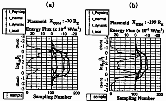
図:イオンのベータ値 ( \beta_i ) で整理したエネルギーフラックス及びその3つの成分。 (a) X_{GSM} \sim -70 R_E での5例のプラズモイドよりなる。 (b) X_{GSM} \sim -199 R_E での4例のプラズモイドよりなる。 データの sampling time は約 12 秒である。縦軸は \log \beta_i であり、 \beta_i \geq 0 の時は図の上半分に、 \beta_i < 0 の時は下半分に分けて示してある。
