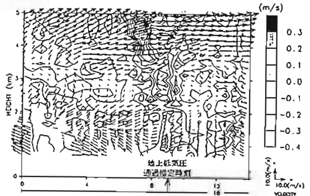
図 1: 1992 年 6 月 18 日の水平風変動 (矢印) と鉛直流動変動 (コンター)。
