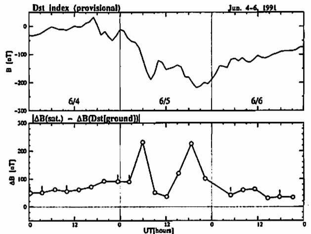
図1 上図: 1991年6月4-6日磁気嵐時のDst-index、下図: 同期間中にあけぼの衛星で観測された全磁力のΔBとDst-indexの差
