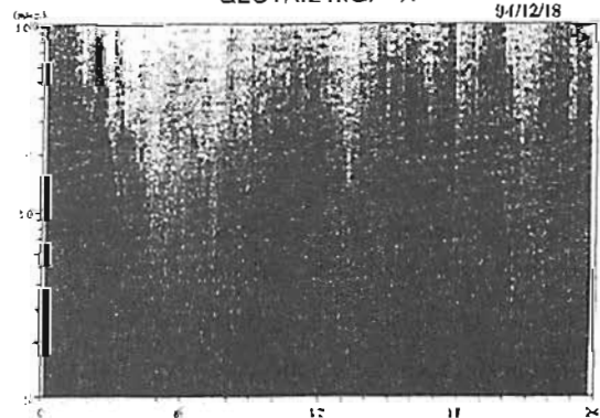
図2 図1の磁場変動 Bx 成分のガイナミックスペクトル
