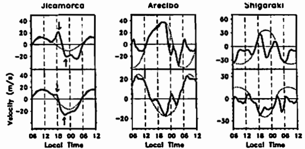
図：地磁気静穏日におけるF領域プラズマドリフト速度の磁力線直交成分。(a) Jicamarcaにおける鉛直上向き成分[中太陽活動期・夏(上)と冬(下)]、(b) Areciboにおける(上)東向き( V_{EL} )および(下)北向き成分( V_{NL} ) [低太陽活動期・夏]、(c) 宿楽における(上) V_{EL} 、(下) V_{NL} [低太陽活動期・夏]。
