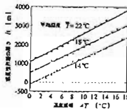
図2 平均気温 T および気温振幅 \Delta T と惑星境界層の厚さ h との関係。これより、実験式として
