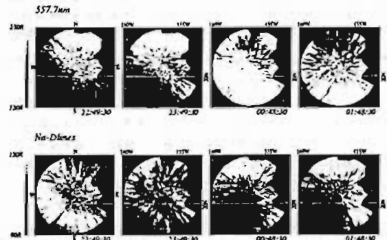
図1 1994年11月5日22時50分から1時50分におけるO1557.7nm大気光とNaD大気光の全天画像の比較。上が北、右が東であり緯線、経線は1度おきにする。
