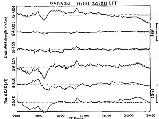
図2 地電位差および磁場の時間変化。上段から有村のNS、EWの地電位差、牛根のNS、EWの地電位差、垂水の磁場のH、D成分。
