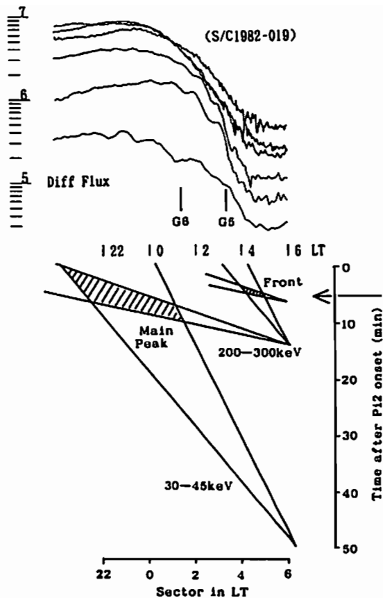
東向きドリフト開始時の電子フラックス経度分布
