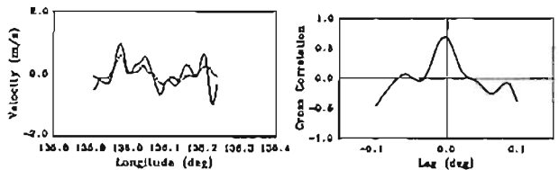
図1: (左) 相互相関の計算に用いたMUレーダーデータ(実線)と航空機データ(破線)。データ間隔は0.001°。前者は位相速度-8.0m/sとして空間データ列への変換を行った。後者はMUレーダー上空を東から西へ飛行した場合のデータである。また、各々約10分~1時間、約2~20kmのフィルクをかけてある。(右) 左図に示したMUレーダーデータと航空機データから計算した相互相関係数。横軸のラグは程度(deg)に相当する。
