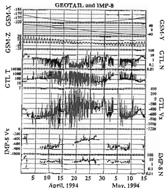
図. 94 年 4 月 1 日から 5 月 15 日に得られた、GEOTAIL の位置 (上)、プラズマ密度・温度・流速 (中) と、IMP-8 で得られた太陽風速度と密度 (下)
