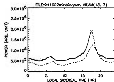
図2. 観測された銀河電波強度の日変化特性(ドット)と30MHzマップから推定される日変化特性(一点鎖線)との比較図。
