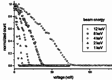
He + ビーム入射時の偏向板を通過する粒子数。横軸は偏向板に印加する電圧を要す。
