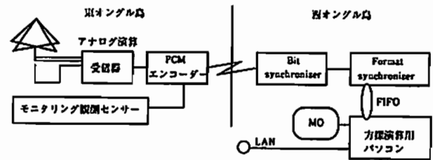
昭和基地VLF方探ブロック図
