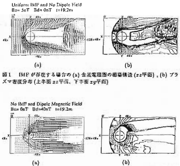
図2 IMFが存在しない場合の(a)水星電磁圏の磁場構造(zx平面),(b)プラズマ密度分布(上半面xz平面、下半面xy平面)
