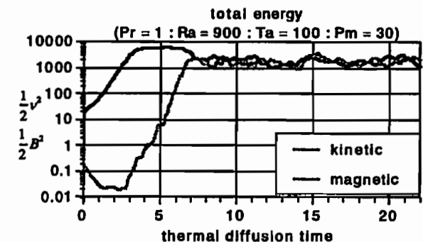
図:全磁場エネルギーと全運動エネルギーの時間発展 (打ち切り次数:4)
