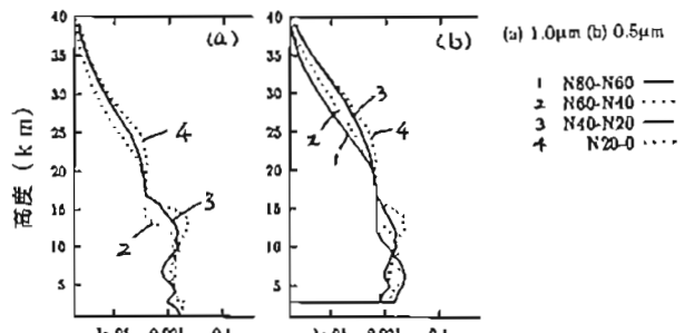
図2 1989年6-8月の0.5μmと1.0μmの消光係数の比の高度・緯度変化
