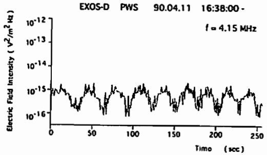
図1 地球ヘクトメートル波に含まれる周期性変動成分
