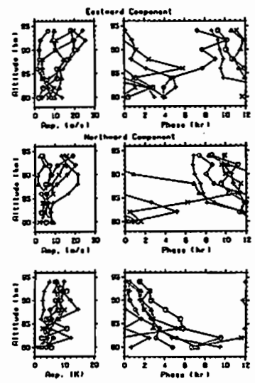
図 MUレーダーを用いた流星観測により冬期に伊奈で観測された半日周期大気潮汐波。上から東西、南北風速および温度変動成分。位相は振幅最大となった地方時を表す。観測される温度変動は時間平均値に対する割合であるのでCIRA1986より背景温度180Kを仮定して絶対値に換算してある。
