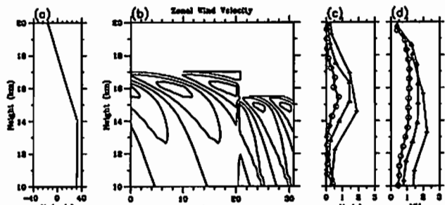
図1. (a) モデル計算で与えた背景東西風速、(b) 東西風速の計算結果、(c)(b)の鉛直ウェーブレット解析結果の平均、および(d)3週間連続観測結果の東西風速のウェーブレット解析結果の平均 ( \lambda_z : ○: ~1 km, Δ: ~2 km, +: ~4 km)。ただし、 c = \omega/k = 4.1 から 13.9 m/s へ変化。波深 ( \alpha_0 = 5 km) での振幅 u_0 = 5 m/s。
