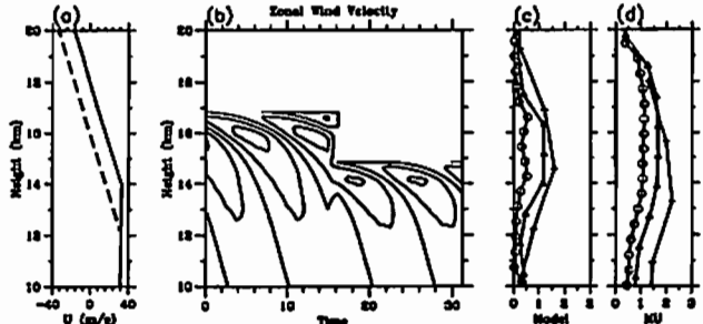
図2. 図1と同様。ただし背景東西風速は実線から破線へ変化、 c = \omega/k = 5.5 m/s で一定の場合。
