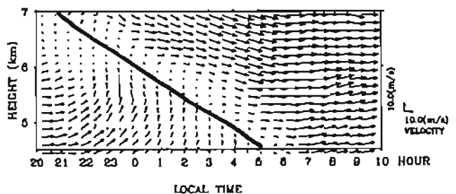
図1 1994年6月22日20~23日10時のMUレーダーによる水平風の時局・高度変化。実線は傾いた前線面を示す。
