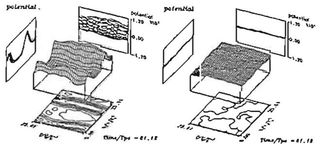
(a) 磁場の強い場合 ( \Omega_e/\Omega_i = 1.0 ) (b) 磁場の弱い場合 ( \Omega_e/\Omega_i = 0.2 )
