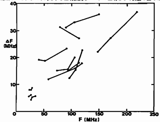
図. ΔF(ω p ) と F(ω p ) の相関関係
