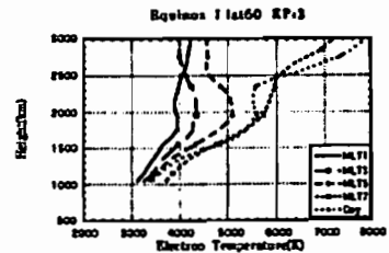
図1: 緯度55~65度の地方時2時間ごとの高度プロファイル
