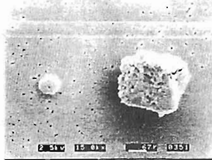
Fig. 圏界面付近(8/25/94: 12.7-11.6km)における、液滴粒子（左）と非球形粒子（右）。この付近では、こうした外部混合状態（それぞれ別々に、非球形粒子の表面は乾いて）していることが多い。
