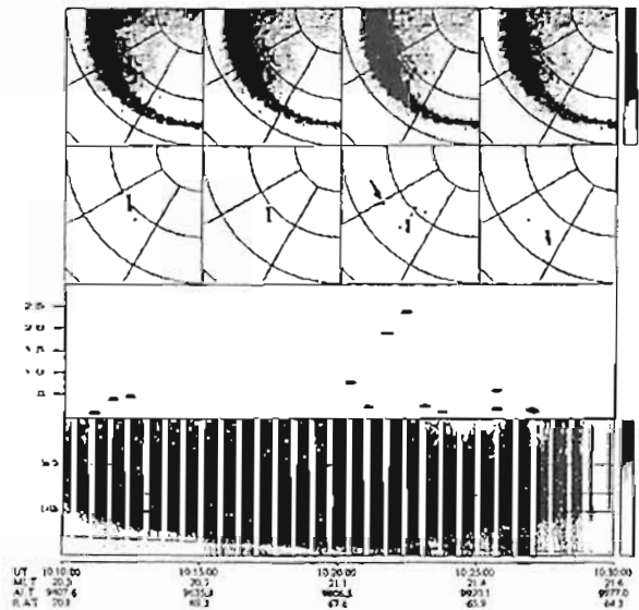
図: 上からATV-UVで撮像されたaurora arc, PWS-PYによるAKR電波源のmapping, 今回おこなった固有値解析による波動各成分の強度比, PWS-DSによるAKR波動のdynamic spectrumを示す。矢印はincoherent AKRの時のmapping。
