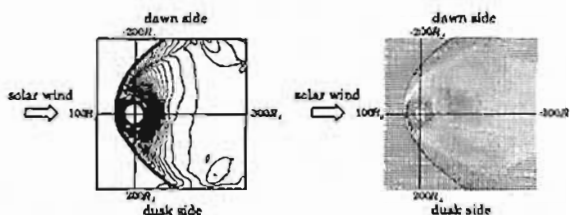
図1. 赤道面における圧力の等高線。図2. 赤道面における速度ベクトル。
