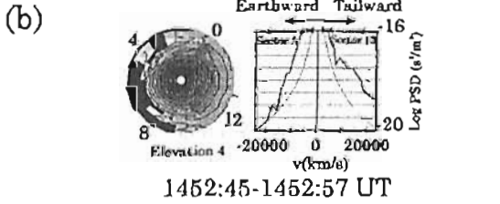
図 (a) 1994年10月2日に観測されたPS-lobe領域のET図 (b) 電子ビームの分布関数
