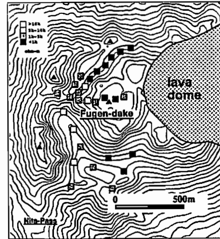
bipole-dipole法によって得られた total apparent resistivityの分布
