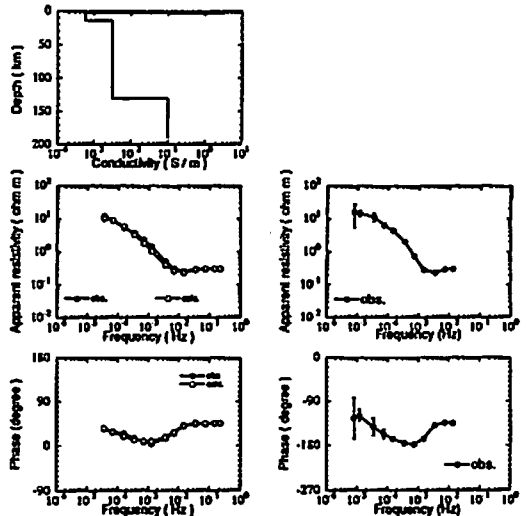
図1 グアム-二宮間の 電気伝導度分布(上)、 見かけ比抵抗(中)、 位相(下)。黒丸は実 測値、白丸は計算値を 表わす。
