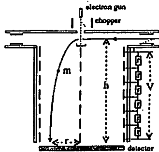
図1. 中性ガス質量分析器概念図 (断面)
