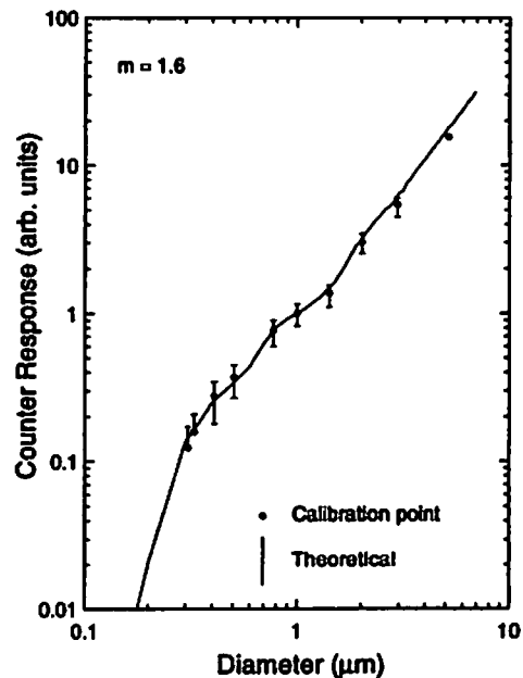
図1 屈折率1.6の標準粒子を用いて行った測定器の校正結果。実線は測定器の光学系その他を考慮にいれた理論計算結果。
