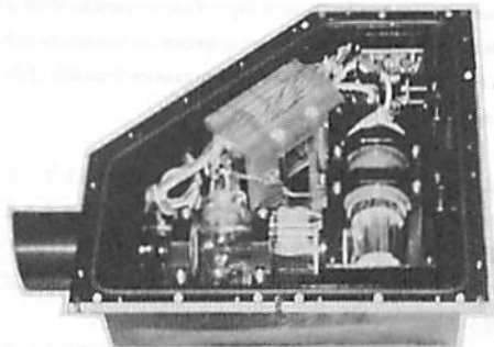
図1 LAPのセンサー部の写真。機軸に対して5.7°(垂直)×42°(平行)の視野を持つ。
