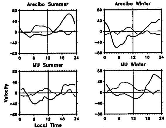
図 1 Arecibo(上)と信楽 MU(下)で観測された太陽活動極大期の夏(左)・冬(右)における V_{E1} (実線) 及び V_{N1} (点線) の平均日変動
