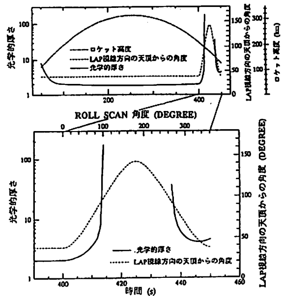
図1. (a) 上から、打ち上げ後の経過時間に対する、ロケット高度・LAP視線方向の天頂角からの角度・光学的厚さの変化。(b) 400-450秒間の拡大図。水平方向を見ると、光学的厚さは増大する。グラフが切れているのは、LAPが地表を見ていることによる。
