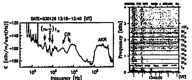
図1 SFAによる電界の周波数スペクトル
