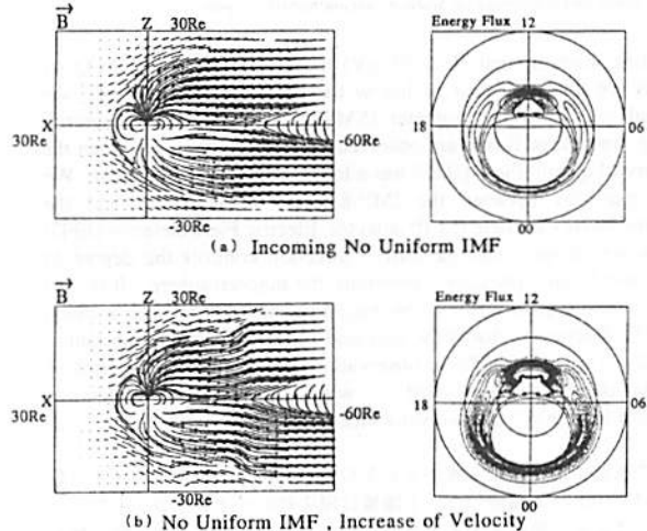
図1 地球磁気圏の磁場構造 (XZ断面図) と Energy Flux 分布 (極冠投影図) (a) V = 300km/s , B_z = 0nT の太陽風を流してから180分後 (変化直前) (b) V = 450km/s に増加してから15分後
