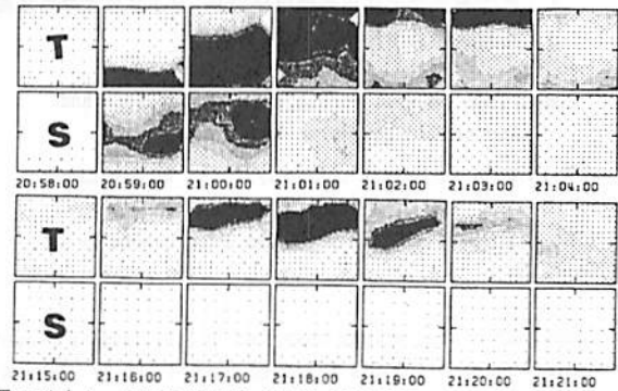
図1a(上) 1993/2/18 2058-2104UT のCNA画像 図1b(下) 1993/2/18 2115-2121UT のCNA画像 Tチョルネス、S昭和 上が高緯度側 右が東側
