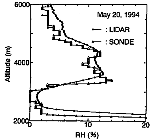
図、ラマンライダー、気象ゾンデにより観測された相対湿度の高度分布。
