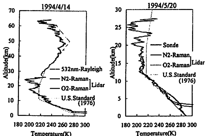
図1. ライダーから求めた気温分布 図2. 気象ゾンデとの同時観測の結果
