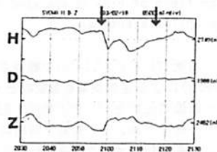
図2 1993/2/18 2030-2130UT の地磁気変化(昭和基地) 500[nT/div]
