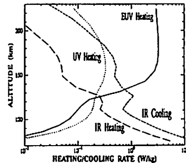
図 1. 緯度 60° における加熱・冷却率
