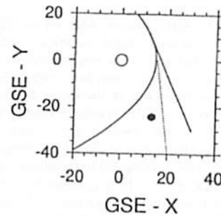
図1 (上) : 1994年6月30日に観測したイオンのEt図。エネルギー散列 (5~40 keV) の時間変化をカウント数/1.2秒サンプルの濃淡表示で示す (カウント数の高低が色の濃淡に対応)。 図2 (下) : 上図 dispersion が観測されたときの配置図。 直線: IMFの向き、点線: foreshock boundary (20 keV) 曲線: 衝撃波の位置、黒点: 衛星の位置。
