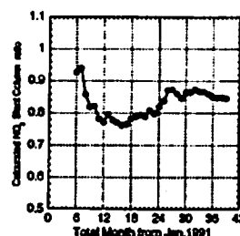
Fig.2 モデル計算による減少率
