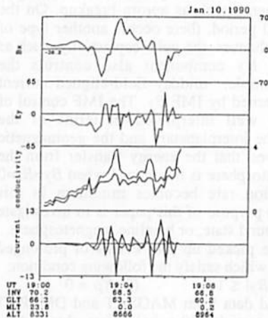
図1 2つの方法で求めた沿磁力線電流変動。上段から磁場の東西成分、電場の南北成分、電離層電気伝導度 (太線: \Sigma_H 、細線: \Sigma_P )、沿磁力線電流密度 (太線: 電場と \Sigma_P から求めた沿磁力線電流、細線: 磁場から求めた沿磁力線電流)
