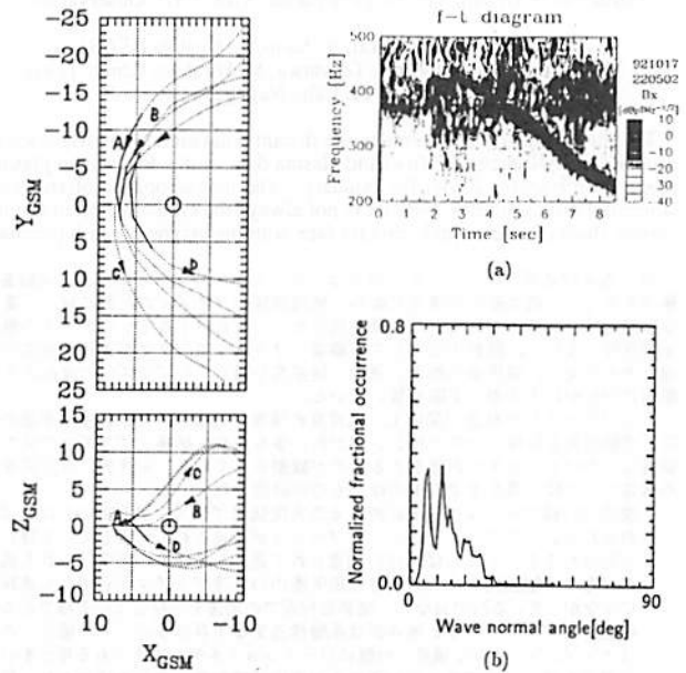
図1 コーラス観測時の GEOTAIL 衛星の軌道。
