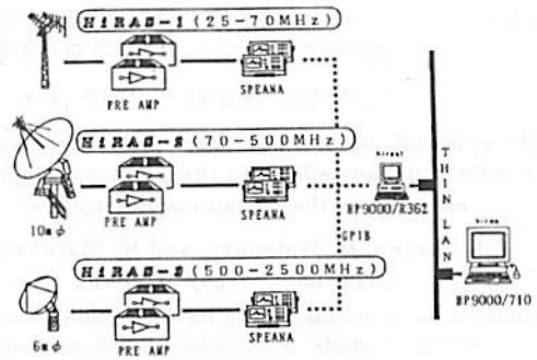
図1. H i R A S (広帯域太陽電波観測装置)
