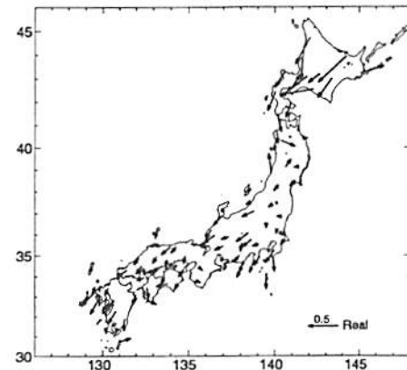
図-1 水平成分の地磁気変換関数の観測値(周期6.4分, 実数部)
