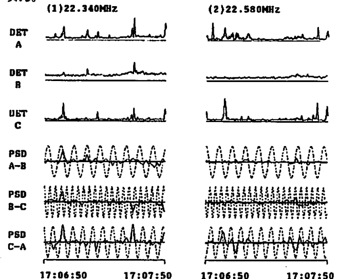
【第1図】1994年7月18日17:6:50から17:7:50 (JST) の干渉計のデータとフリッジに計算値。上から順に川波 (A)、蔵王 (B)、米山 (C) の強度データ、A-B、B-C、C-Aの干渉波形、木星フリッジの計算値をしめす。(1)、(2)はそれぞれ、22.340MHz、22.580MHzのデータである。
