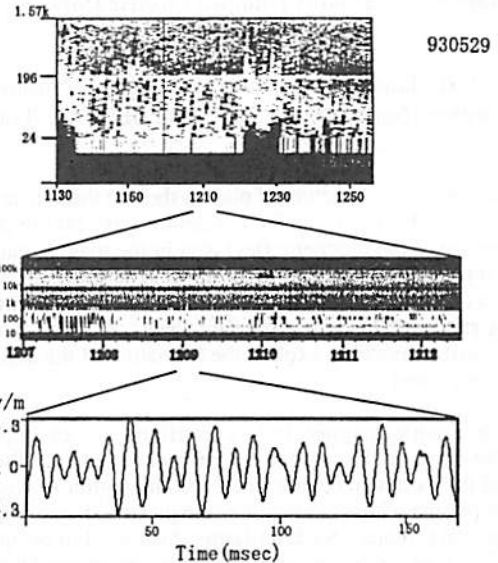
図1: SFA, MCA, WFCからみた狭帯域静電波
