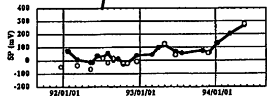
図1: 1992年以降の自然電位変動(雲見岳・仁田前)。代表的な2点を選んで示した
