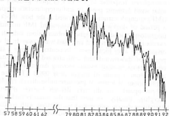
図1 棒間の磁場H成分の月平均値グラフ。細い線がDst<-15の日を除く前、太い線が除いた後のものである。横軸の1目盛りは1年、縦軸の1目盛りは10nTに当たる。
