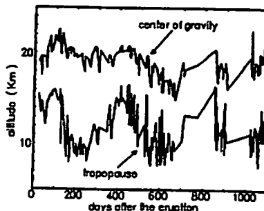
Fig.2 後方散乱係数の重心と圏界面の高度
