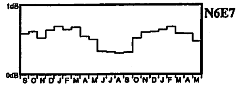
図3 QDCの平均レベルの月変化(N6E7方向)
