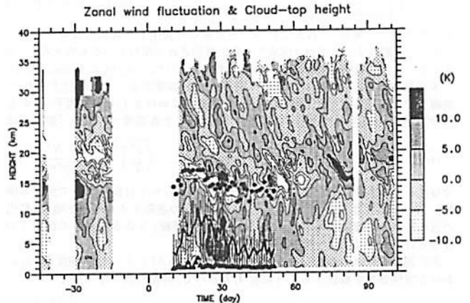
図 東西風に4日以上ローパスフィルターをかけたものの時間高度断面にバンドン周辺の積雲の最高高度(○)、平均高度(太線)を重ねて描いたもの。横軸は93年1月1日を1とした日数。
