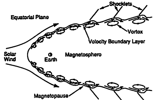
図2. Miura (1992) のローカルなシミュレーションに基づく、赤道面内でのグローバルな K-H 不安定の描像。矢印は流れの向きを表す。
