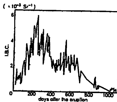
Fig.1 後方散乱係数の積算値 (I.B.C.)
