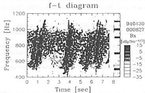
図1 1993年4月30日に観測された Rising tone のダイナミックスペクトル
