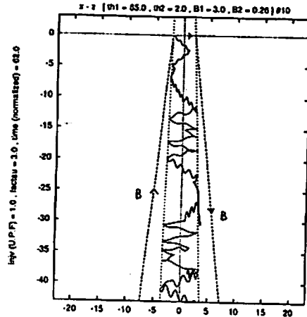
Fig.1 Shock angle \Psi_1 = 85^\circ , \Psi_2 = 2^\circ の対称な slow shock pair 中に上流から injectされた粒子の軌道。外側の2本の点線は磁力線を変わり、その内側の点線は2枚の slow shock を示している。粒子は、bulk flow に流されながら衝撃波を横切ったり散乱を受けたりし、その度に pitch angle と gyro-phase angle が変化する。粒子のエネルギー変化は、衝撃波をきるとき curvature drift (加速) と gradient B drift (減速) の大小関係によって決まり、上流から下流にぬける粒子は、そのときの pitch angle によって減速、または加速を受け、下流でミラー反射される粒子は常に減速、また下流から上流にぬける粒子は常に加速を受ける。従って、粒子が加速される為には、上流で散乱されて pitch angle や gyro-phase angle が変化を受ける必要がある。
