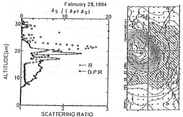
2月28日の成層圏エアロゾル観測結果(エアロゾルの後方散乱係数Rと偏光率D.P.R.) 及び、測定気圧偏風成分(30hPa)
