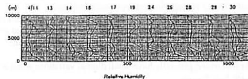
図1. 1994年4月の名古屋のラマンライダーと浜松のゾンデで観測された湿度
