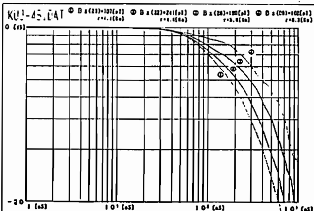
図2 磁場B z 成分の減衰曲線(冬化) 送信機から4.1km (○), 4.8km (◇), 5.6km (◎), 6.3km (⊙) 離れた地点でのデータ。約20msパルス長、送信電流32A
