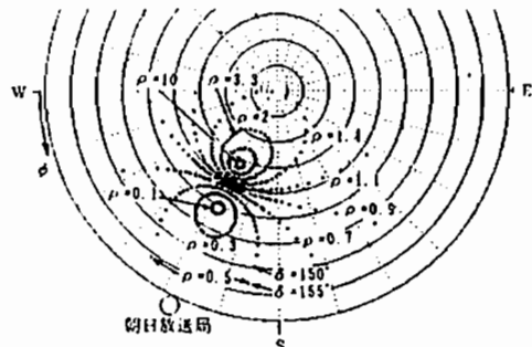
図2 E s 層と F 層反射波が混在したときの理論的方向探知機が示す到来方向
