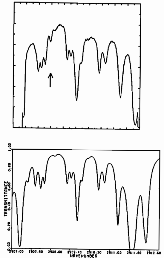
図. 測定スペクトル(上)と合成スペクトル(下)の比較 2908.53 \text{cm}^{-1} に未同定線がある。
