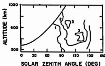
図1. Pioneer Venusによって観測された昼側から夜側へのO+の水平方向の平均速度(km/s)。左上の境界はionopauseの平均的位置を示す [Miller and Knudsen, 1987]。
