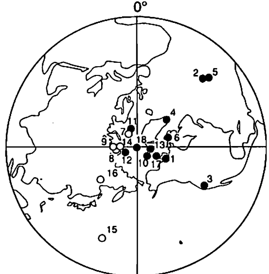
fig.2 安定磁化方向より求めたVGP。
