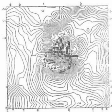
図2 磁気異常図 (コンターマップ)
