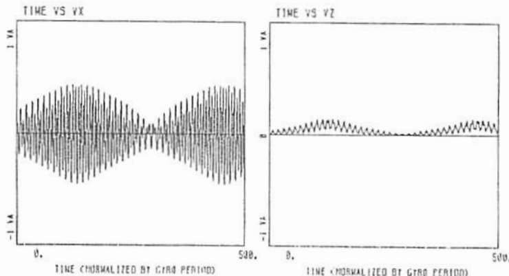
図1. 斜め伝搬 (60°) するアルフベソ波によるイオンの加速。波の周波数がイオン・サイクロトロン周波数の1/1.9のところで起きた低調波共鳴による。(左): 平均磁場に垂直な速度成分の時間変動 ( 0 < \Omega_{it} < 500 )。縦軸はアルフベソ速度で規格化してある。速度が0.4 VA程度で頭打ちになっているのは非線型過程の飽和による。(右): 平均磁場に平行な速度成分の時間変動。斜め伝搬波による加速ではイオンは磁場に平行にも加速される。
