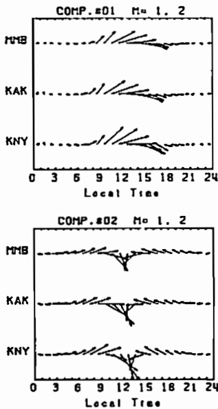
図1 冬の主成分固有ベクトル(第1, 2主成分)。ただし90度回転して等価電流ベクトルとして表現している。
