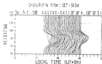
図4 フィルタリングプロファイル(長波長域)
