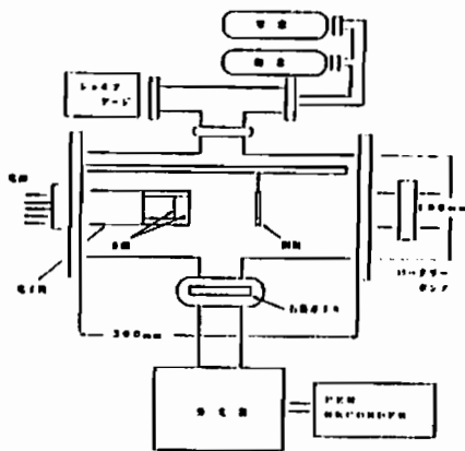
図 1. 実験装置
