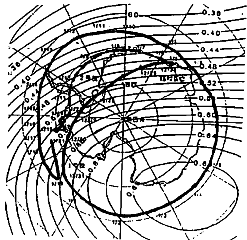
図1 PPBの航跡と全磁力(IGRF)
