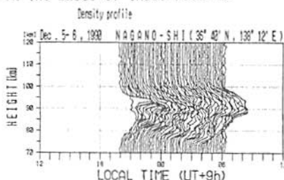
図1 ナトリウム原子密度プロファイル
