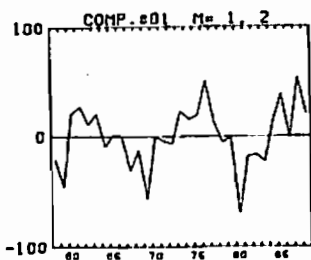
図2 冬の第1主成分量の長期変動。
