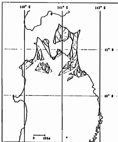
図：観測網内の三角区域。各区域内でインピーダンステンソルを求める。*は水沢測地観測所。
