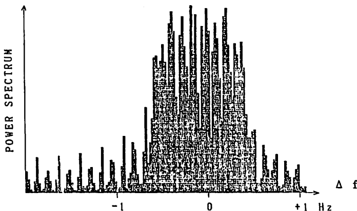
図 サンプル時間内に反射点に変化した場合の ドップラースペクトルのシミュレーション結果
