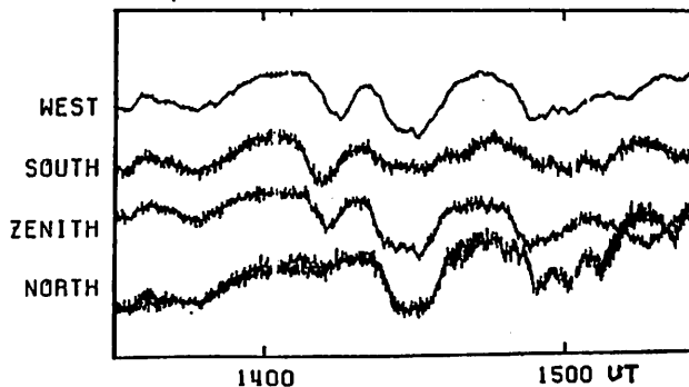
図3 CNA領域の磁南から磁北への移動
