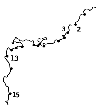
第2図 変砂鉄採取地点(長門北浦海岸)
