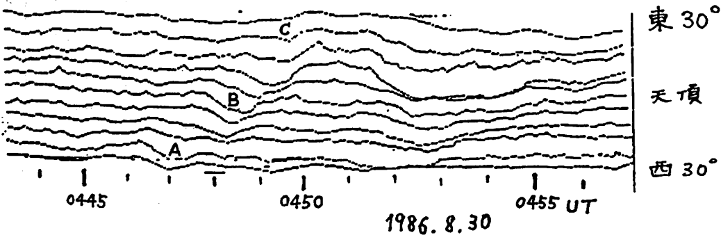
図 1 東西掃引ビームによる、pre-dawn の CNA 脈動。
