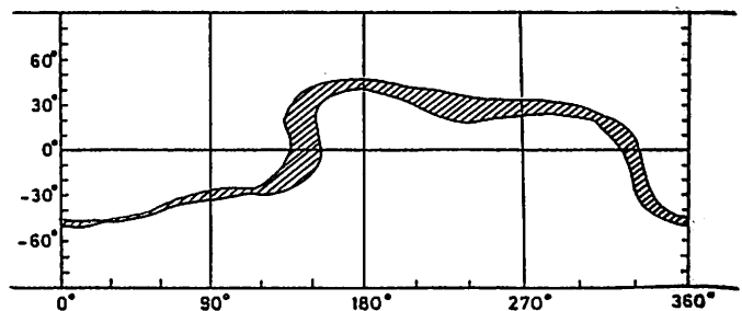
図4. ソースサーフェイス上の磁気中性線
