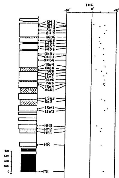
図3. 31ヶ所のサイトの縦断上での位置関係と磁化傾向。
