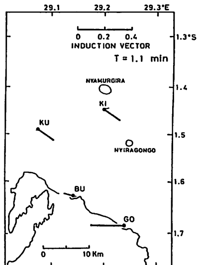
同期63分(左)と1.1分(右)の Transfer ft. からの求めた Induction arrow. 太線一実部、細線一虚部
