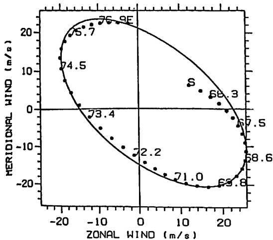
図1 1986年10月20日9～11時の平均風速のホドグラム。●は平均風速に6～24 kmを通過域とするバンドパスフィルターを施して得られた値。実線は観測値に楕円をフィッティングした結果を示す。図中の数字は高度(km)を示す。
