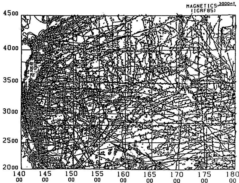
図1 北西太平洋の地磁気異常のProfile図
