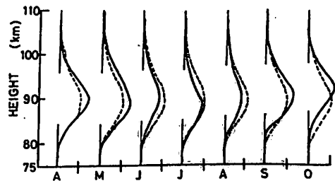
Fig. 2, 月別高度分布（点線、全平均）
