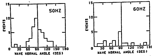
図1. 電力線放射が観測されたときのアンテナと磁力線とのなす角度
