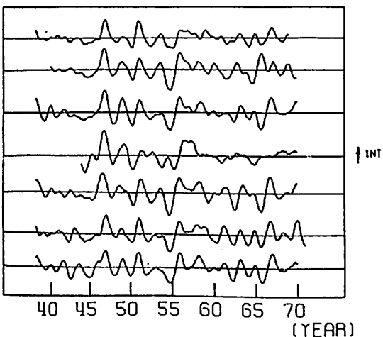
図1 地磁気日変化振幅の準2年周期振動 (上: H成分, 下: D成分)
