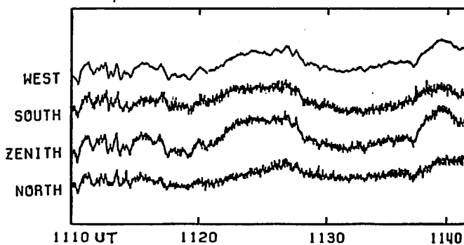
図2. 空間的に均一なCNA
