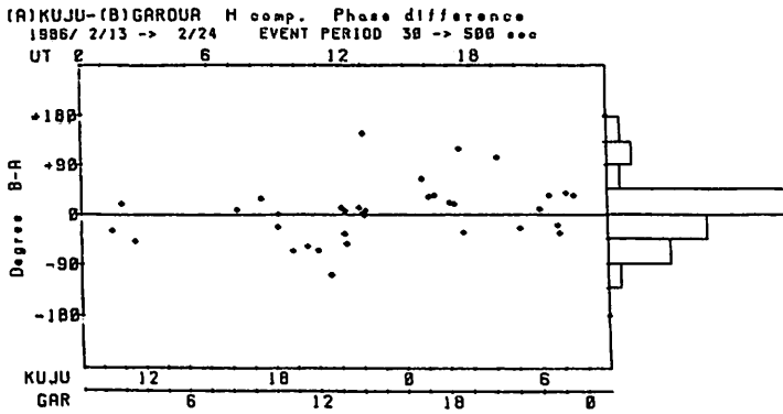
図2': H成分の位相差。右端の分布に注意。分散はD成分より小さい。 久住-ガロワ(アフリカ)-ワンカヨ(ペルー)間。
