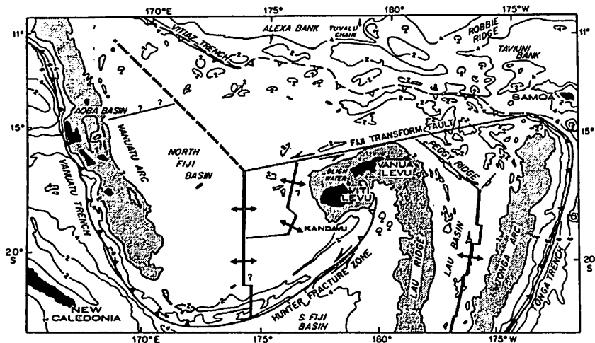
Fiji の位置 after Brocher and Holmes (1985)
