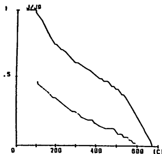
第2図 輝緑岩の J_s -T 曲線
