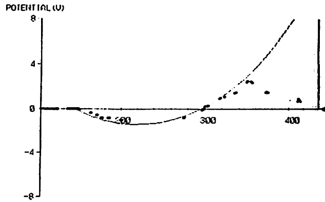
第1図 VxB起電力の計算値(実線)と計測値(点)
