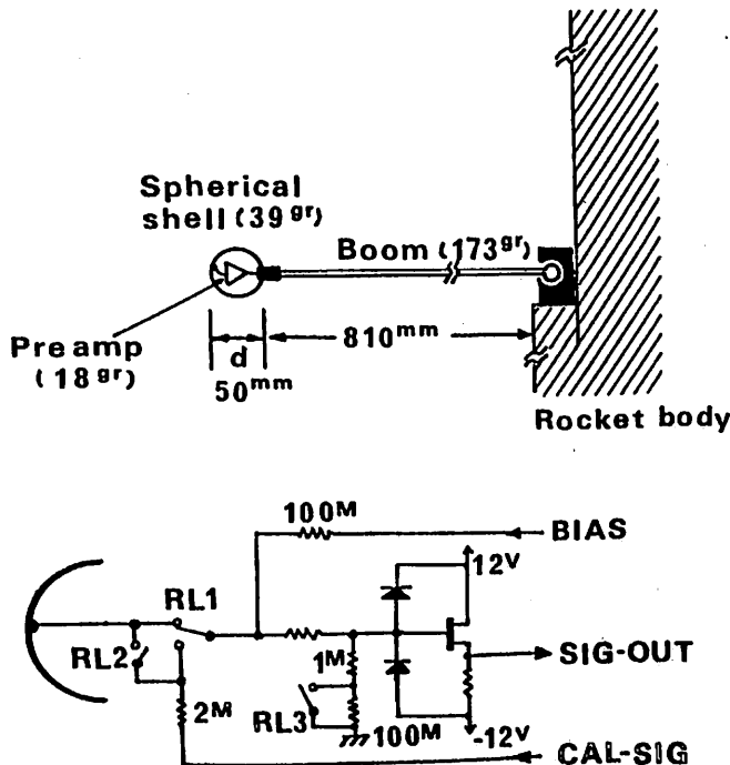
図 1 球プローブの概念図 (上) 右左対称であり左側のみ示してある。BOOMは5mmφの真ちゅうパイプで内部に電源ラインや信号ラインが通っている。BOOM自体は Rocket Body と同電位である。球殻は BOOM と絶縁されている。 (下) 図に記されている回路図は、観測モードとして、信号ドレイブ用の OPAMP 1 ケ、電源ノイズカットフィルタがある。
