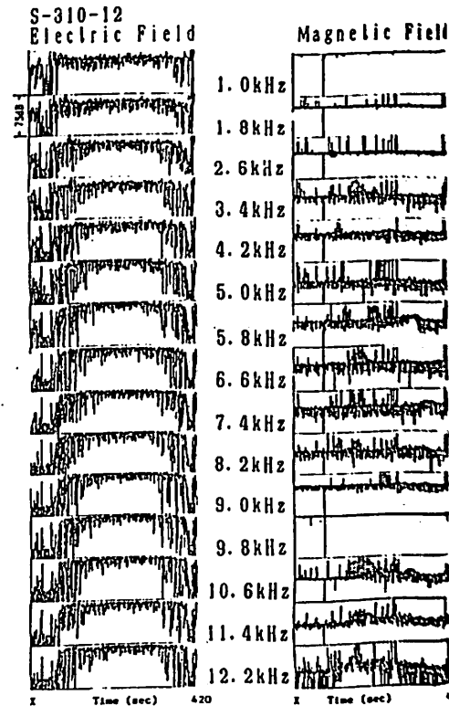
図1 S-310-12号機におけるSFRで測定した電界及び磁界成分
