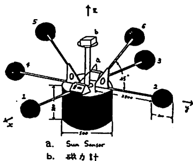
図1 観測器概略図
