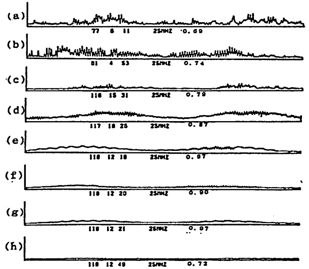
図1 25MHz帯での木星方向からの電波 端から端までが1周期 いずれも1978年最初の数字は、DAY OF YEARを 2、3番目は、時刻を最後に、相関係数を表す
