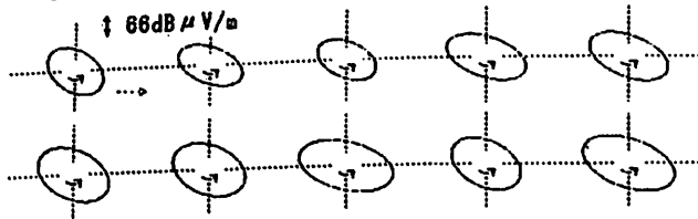
図3 ニッポン放送の観測例('87年1月8日)
