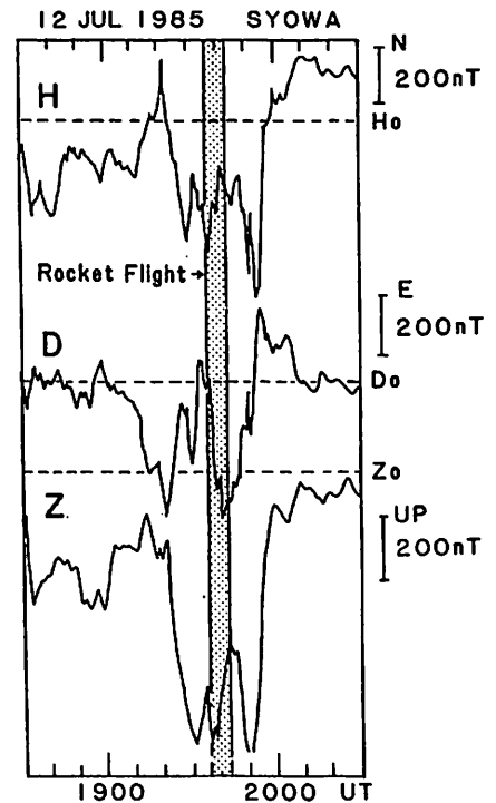
図1 ロケット飛行時の昭和基地マグネトグラム
