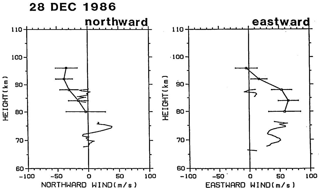
図1 流星観測と乱流散乱観測で得られた風速の高度プロファイルの比較
