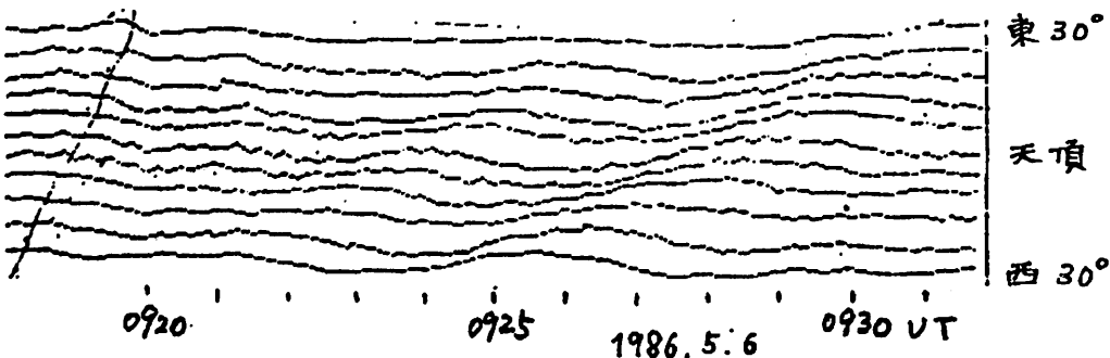
図 2 morning に発生した CNA 脈動。周期 4 分、速度は東向 300m/s
