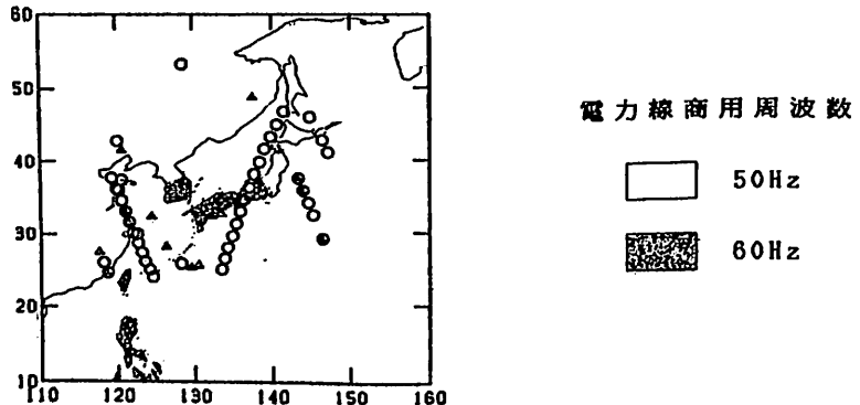
図2. 電力線放射の位置分布(50Hz○印、60Hz△印)と地上の電力線商用周波数
