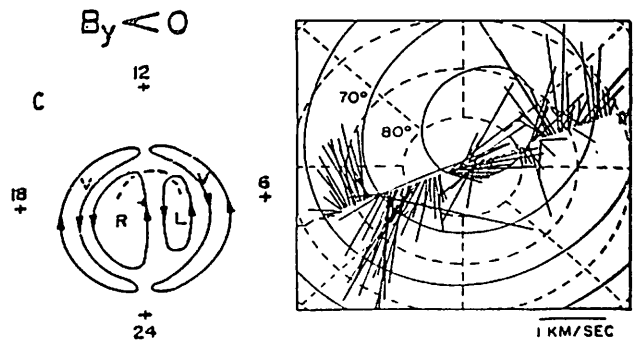
図2 (左) Reiff et al. (1985) によって提案された対流モデル Lはlobe cell, Rはreclosure cellを表す。 (右) \ominus オーロラ時に観測されたイオンドリフト (Frank et al. 1986.)
