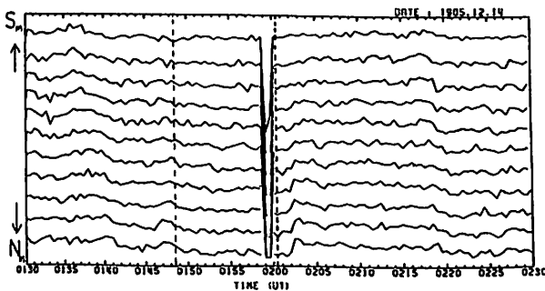
図.2(下) マルチビームリオメータの吸収タイムプロファイル(吸収は上向き)破線はX線計数率のピークを示している。
