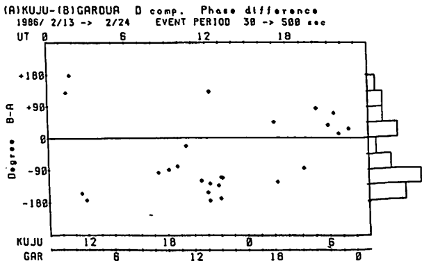
図1': D成分の位相差。右端の分布に注意。分散はH成分より大きい。 久住-ガロワ(アフリカ)-ワンカヨ(ペルー)間。
