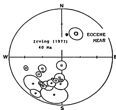
各サイトの平均の磁化方向を \alpha_{95} の円で共にシュミットネットに示す。黒丸は下半球、白丸は上半球への投影を示す。 ○□: 始新世 (□: 傾動補正後) ☆: 中新世 ⊙: 始新世平均 (正帯磁) * : 40MaのVGP (Irving 1977) から求めた石垣島での磁場の方向
