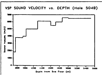
3: VSP レコードと岩石試料の物性。
