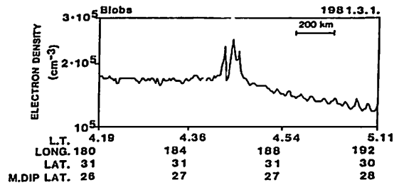
図1. 「ひのとり」衛星によって観測されたプラズマ・ブロップの1例。
