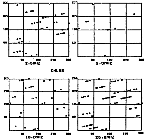
図2 RANのデータを木星の位相(横)とイオの位相(縦)で表したもの 木星の位相は、1965モデル
