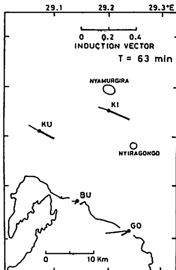
同期63分(左)と1.1分(右)の Transfer ft. からの求めた Induction arrow. 太線一実部、細線一虚部
