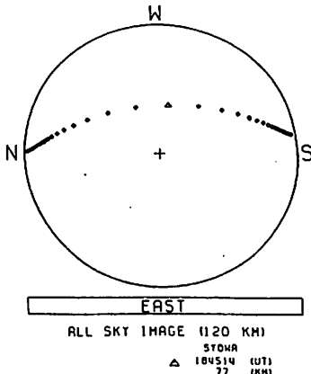
第1図 1983年5月17日 18時45分における、昭和基地全天カメラ及びNOAA衛星同時観測例
