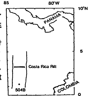
1: Hole 504B 位置図。
