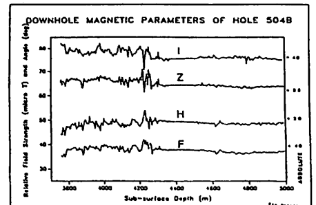
4: BHM による全磁力異常分布断面。
