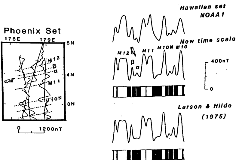
(図1) Phoenix磁気異常群中に新たに発見されたevent
