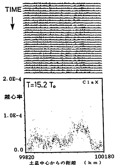
図3. 粒子の動径方向分布と離心率分布
