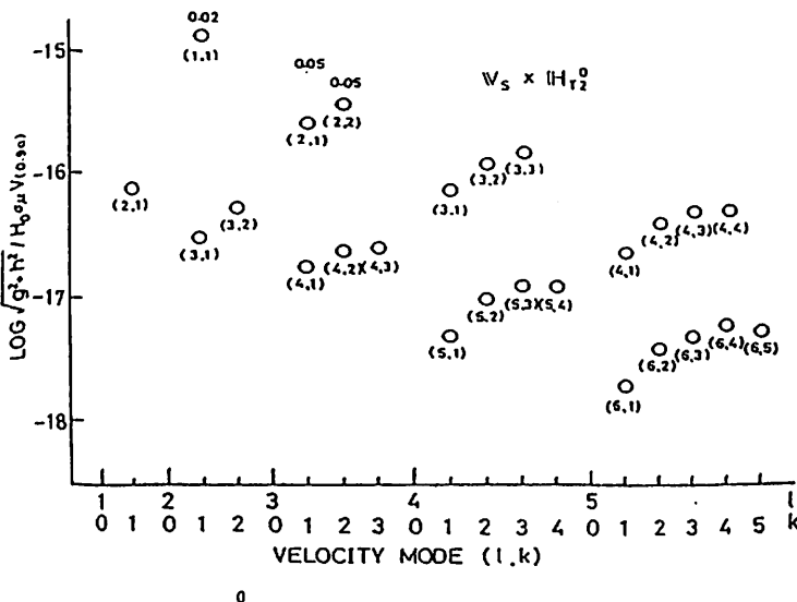
図1: V_S \times HT_2 のつくるポロイダル誘導磁場の強さプロットの上の数字は、二つの磁場の比を表す。
