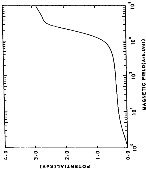
図1 ポテンシャルの1例。 左端がプラズマシート、 右端が電離層。
