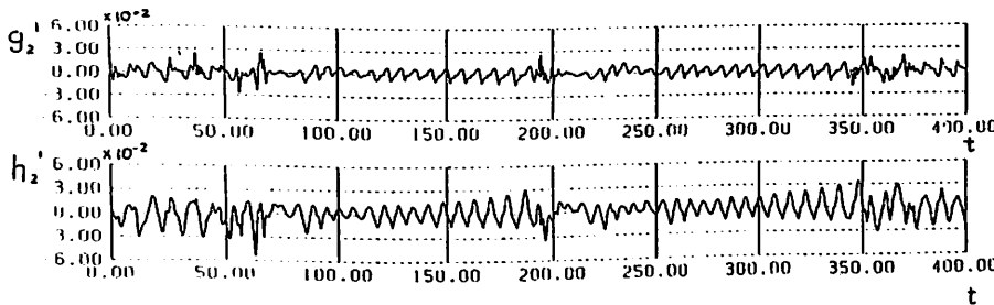
図2 Gauss係数 g_2' 、 h_2' の変動
