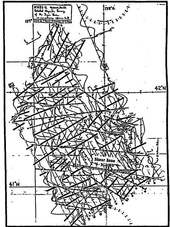
図2) 磁気異常プロファイルと磁気縞模様解釈図 実線: 磁気縞模様。 破線: pseudofault
