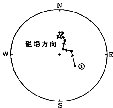
図1. 1インチ角試料(No.11)の磁化方向の時間的変化をシュミット等積投影法にて表した。時間と共に☆の磁場方向へ動くのがわかる。
