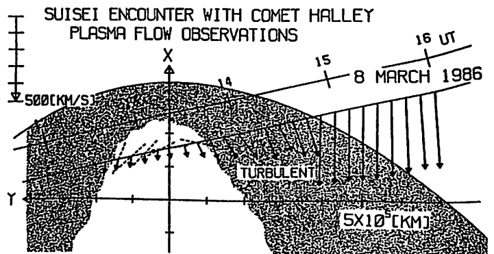
「すいせい」最接近時のプラズマの流れと磁力線方向
