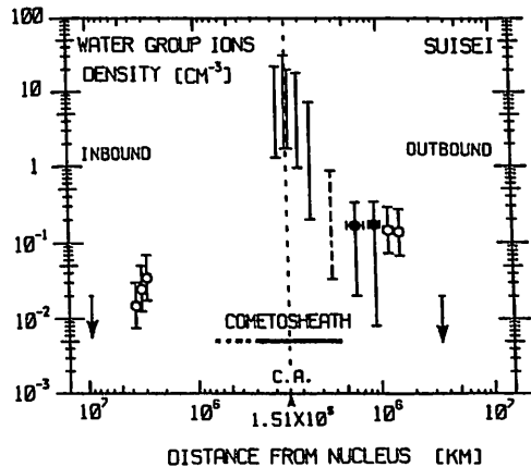
ハレー彗星起源のプロトン(左図)及び水分子族イオン(右図)の空間分布 (注: 横軸のスケールは左図が linear, 右図は Log である)
