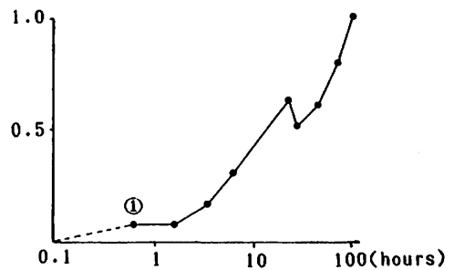
図2. 試料(No.11)の磁化強度の時間的変化。縦軸は磁化強度を横軸は時間(対数)を示す。時間と共に強度は増加している。
