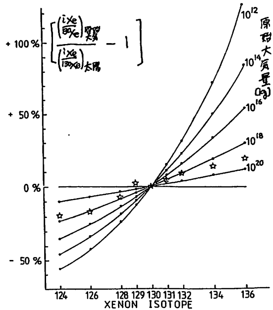
図2. 計算されたXeのfractionation pattern. ☆印は現在の地球大気の数値
