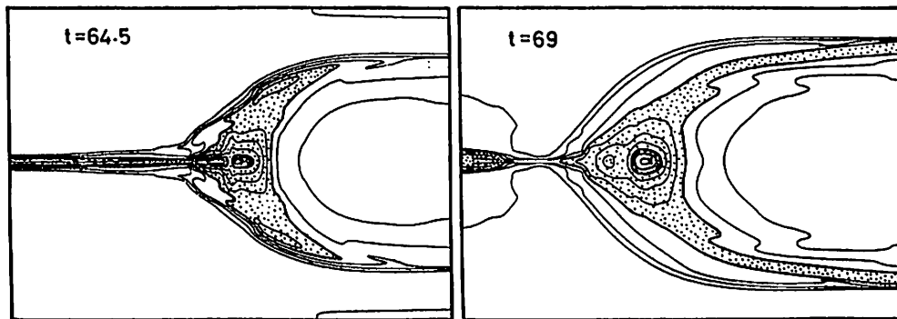
図. 1. 温度 T (\equiv P/\rho) の分布。ドットをつけた領域は温度が約5倍以上、影をつけた領域では10倍以上加熱された事を示す。
