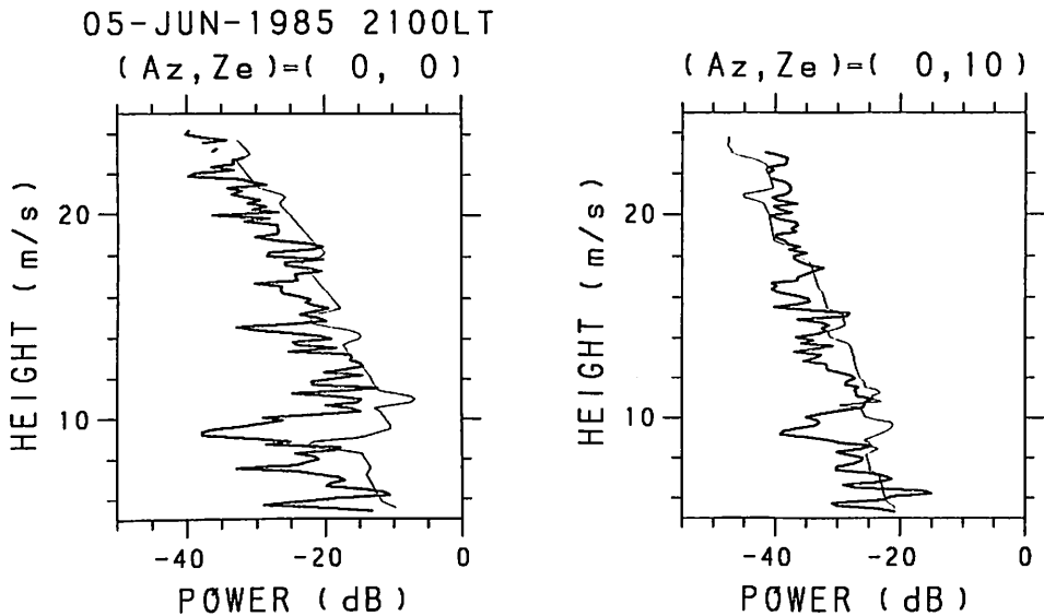
図1 天頂方向(左)と天頂角10度方向のビーム(右)のエコー強度の高度プロファイル。距離による減衰を補正してある。何れも細線はゾンデのデータより求めた理論値。
