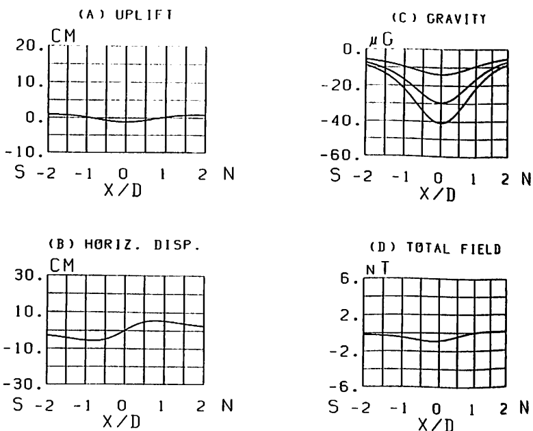
第2図 複合T11クラック・モデル (クラック走向に平行なプロファイル)
