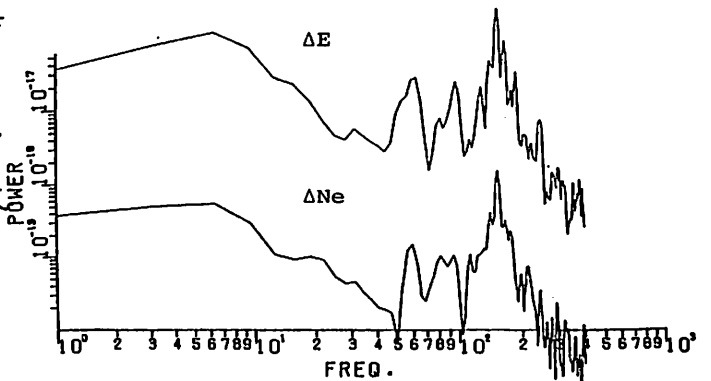
図2. 電場( \Delta E )及び密度( \Delta Ne )ゆらぎスペクトル
