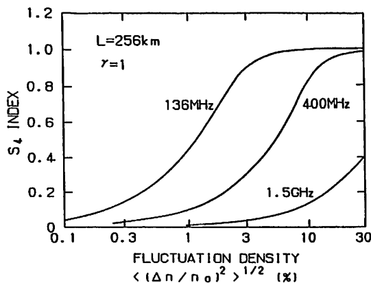
図. S4指数のゆらぎの強さ依存性。3周波数について示す。ゆらぎの厚さは256km、等方的なゆらぎを仮定。
