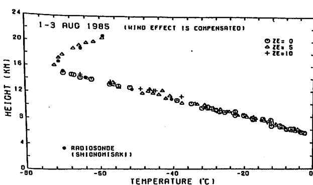
図1 昭和60年8月1～3日の実験により測定された気温高度分布
