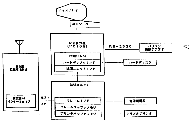
観測装置
