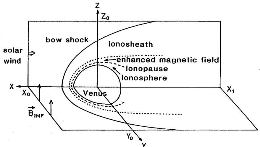
第1図. 太陽風と金星電離圏の相互作用の三次元MHDシミュレーションにおける座標系、金星電離層に惑星間磁場を伴った太陽風が衝突する。
