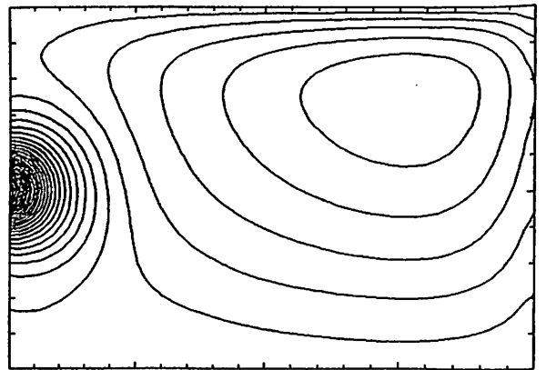
Fig. 3 ( \phi_{||} の等高線)
