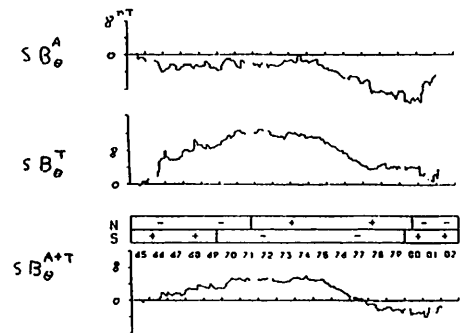
図2 IMF南北成分の長期変動 SB_\theta = \sum_{k=1}^n B_{\theta k}
