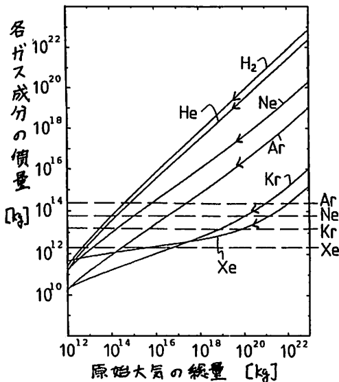
図1. 原始大気散逸にともなう各ガス成分の量の変化。初期大気量 1 \times 10^{23} kg EUV fluxは現在の100倍。水平破線は各希ガス成分の現在大気中の存在量。
