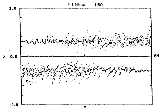
図-1 1次元電子プラズマ系で両端から速度 Vd の冷たいビームを注入し、つづけた時の熱化の様子。イオンは限りなく重いとしてバックグラウンドにはりつけてある。メッシュの数は 64 粒子数: 2000 Vd = 8.0 \omega_p \Delta x で実験開始から 150 / \omega_p たって定常状態に達したと思われるときの x-v 位相空間での粒子分布のプロット。
