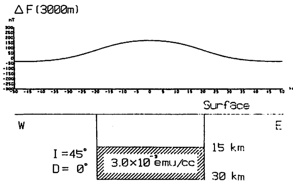
第3図 第2図のデータから求まる見掛け上の磁気構造
