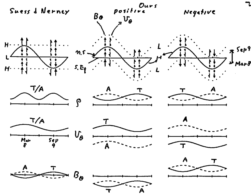
図1 B_\theta, U_\theta, \rho の緯度分布
