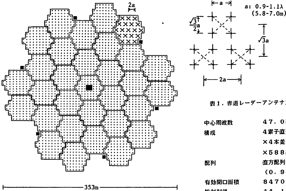
図 1. アンテナ配列。個々の十字は4素子直交八木アンテナを表す。
