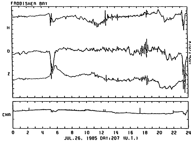
図 Frobisher Bay における波形出力と H 成分のダイナミクススペクトル例
